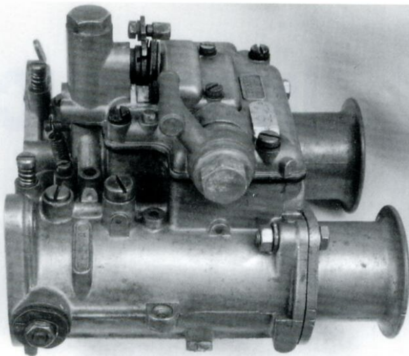
40 DHLA Dellorto.
