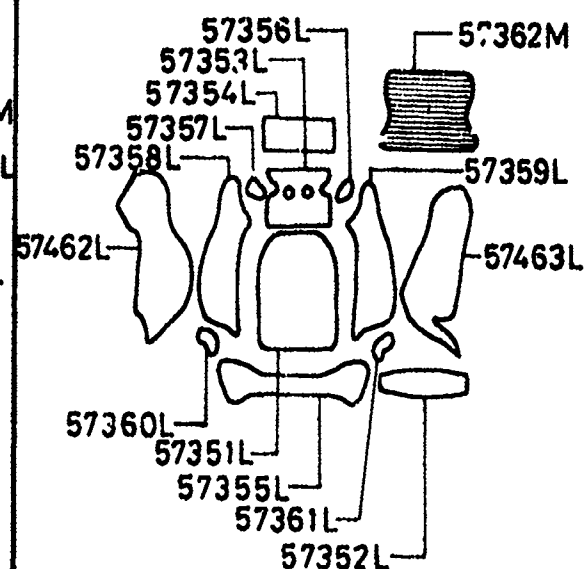
TRIM(L), BACK
