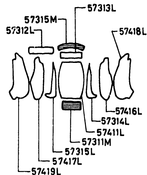
TRIM(L), CUSHION
