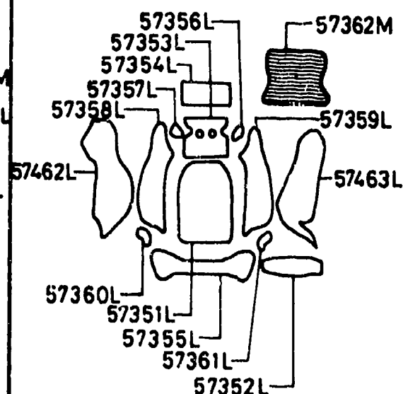
TRIM(L), BACK
